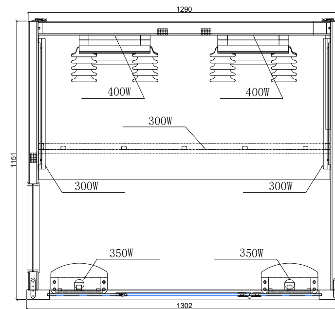
Draufsicht
