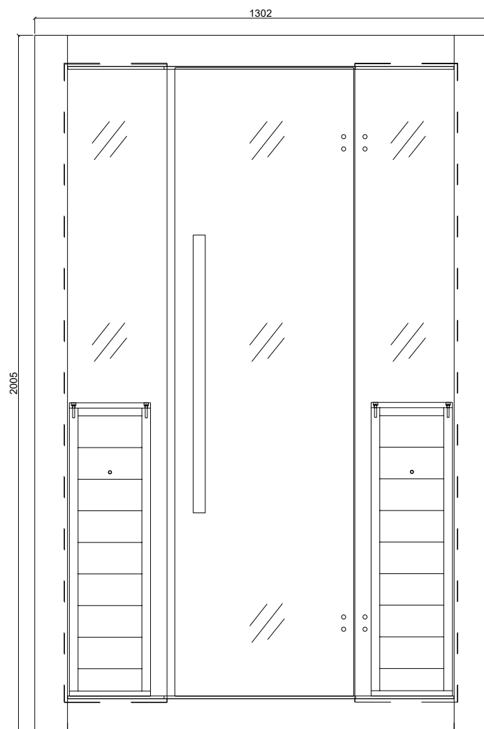
Vorderansicht
