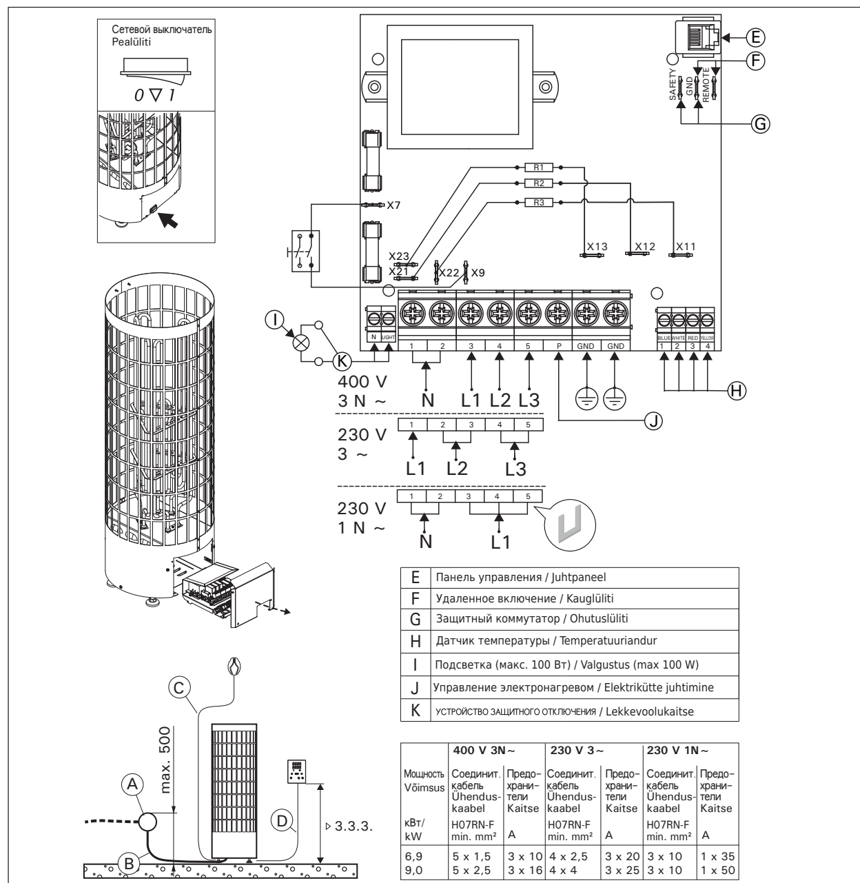
Рисунок 7. Электромонтаж Joonis 7. Elektrihendused
