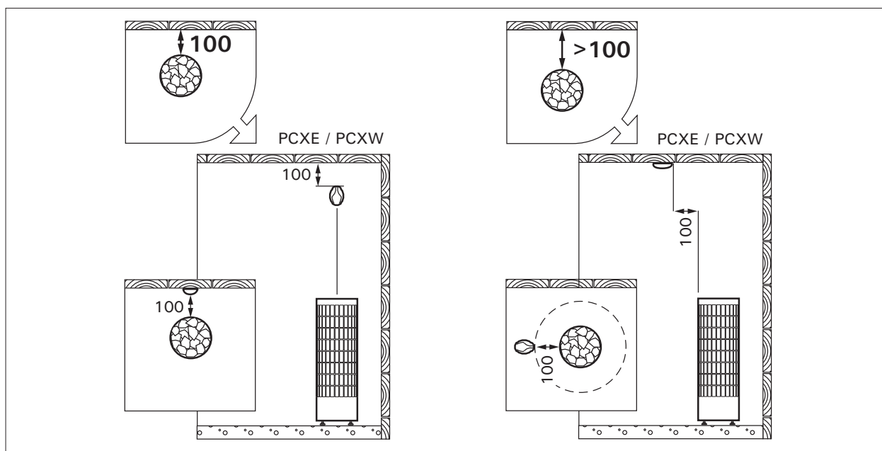
Figure 8. Installation du capteur (toutes les dimensions sont fournies en millimètres) Rys. 8. Instalowanie czujników (wymiały w milimetrach)
