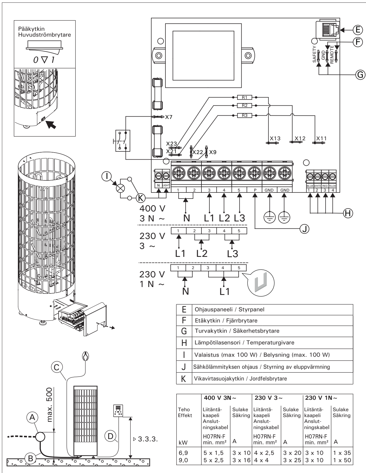
Kuva 7. Sähkökytkennät Bild 7. Elinstallationer
