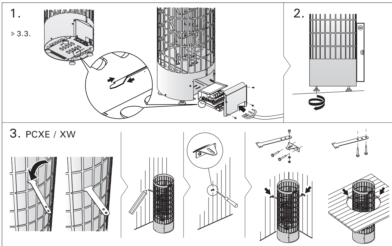
Figure 10. Installing the heater Abbildung 10. Installation des Saunaofens
