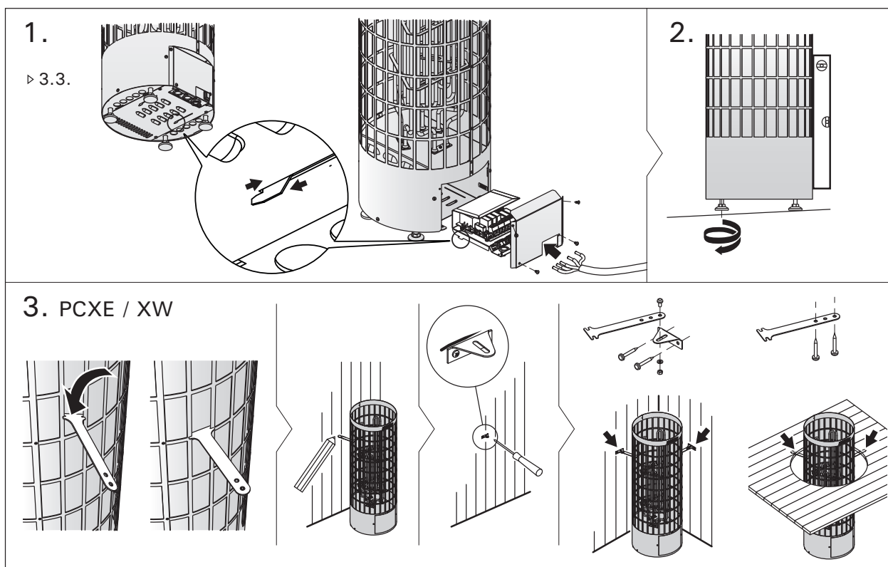
Figure 10. Installation du poêle Rys. 10. Montaż pieca
