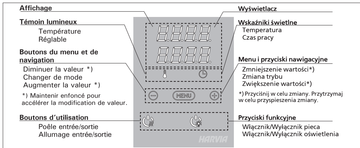
Figure 2. Le tableau de commande Rysunek 2. Panel sterowania
