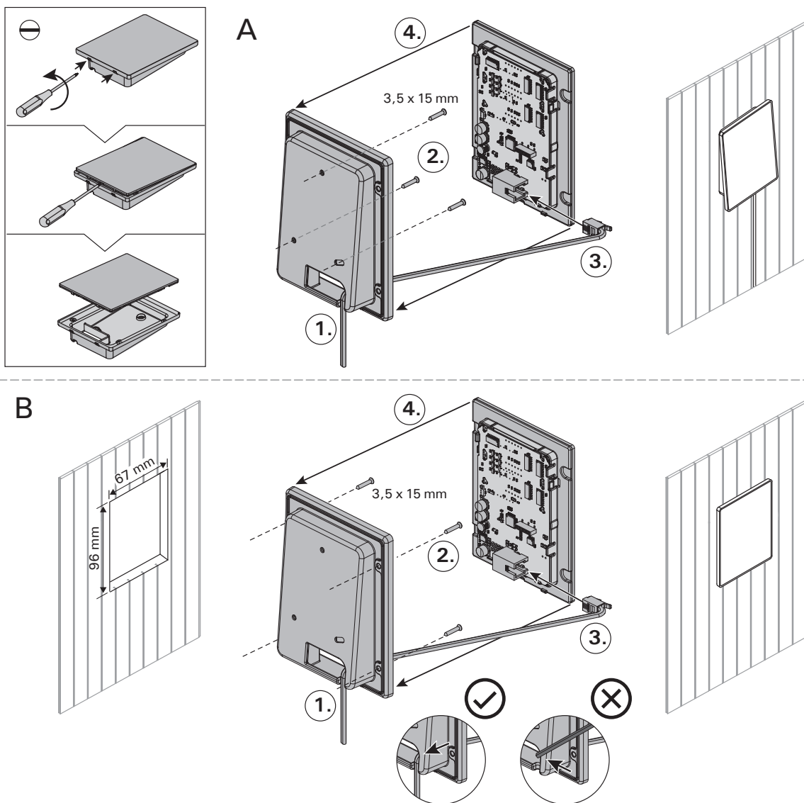
Figure 9. Fixation du tableau de commande Rysunek 9. Montaż panela sterującego
