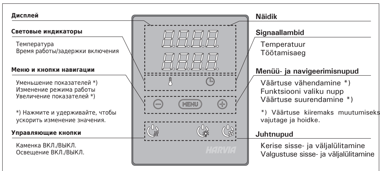
Рисунок 2. Панель управления Joonis 2. Juhtpaneel
