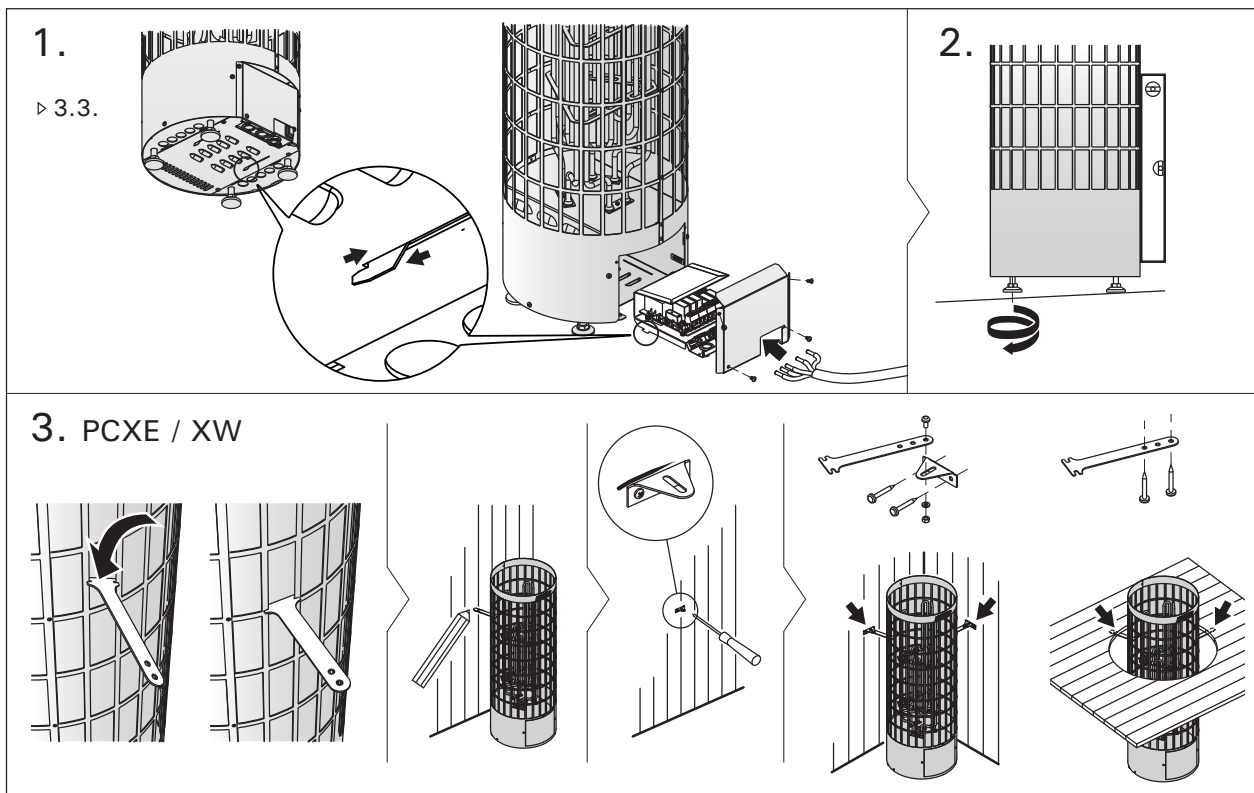
Kuva 10. Kiukaan asentaminen Bild 10. Montering av aggregatet
