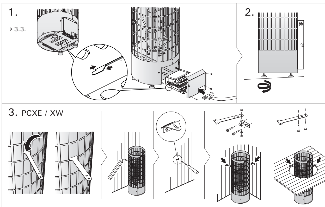
Рисунок 10. Установка каменки Joonis 10. Kerise paigaldamine
