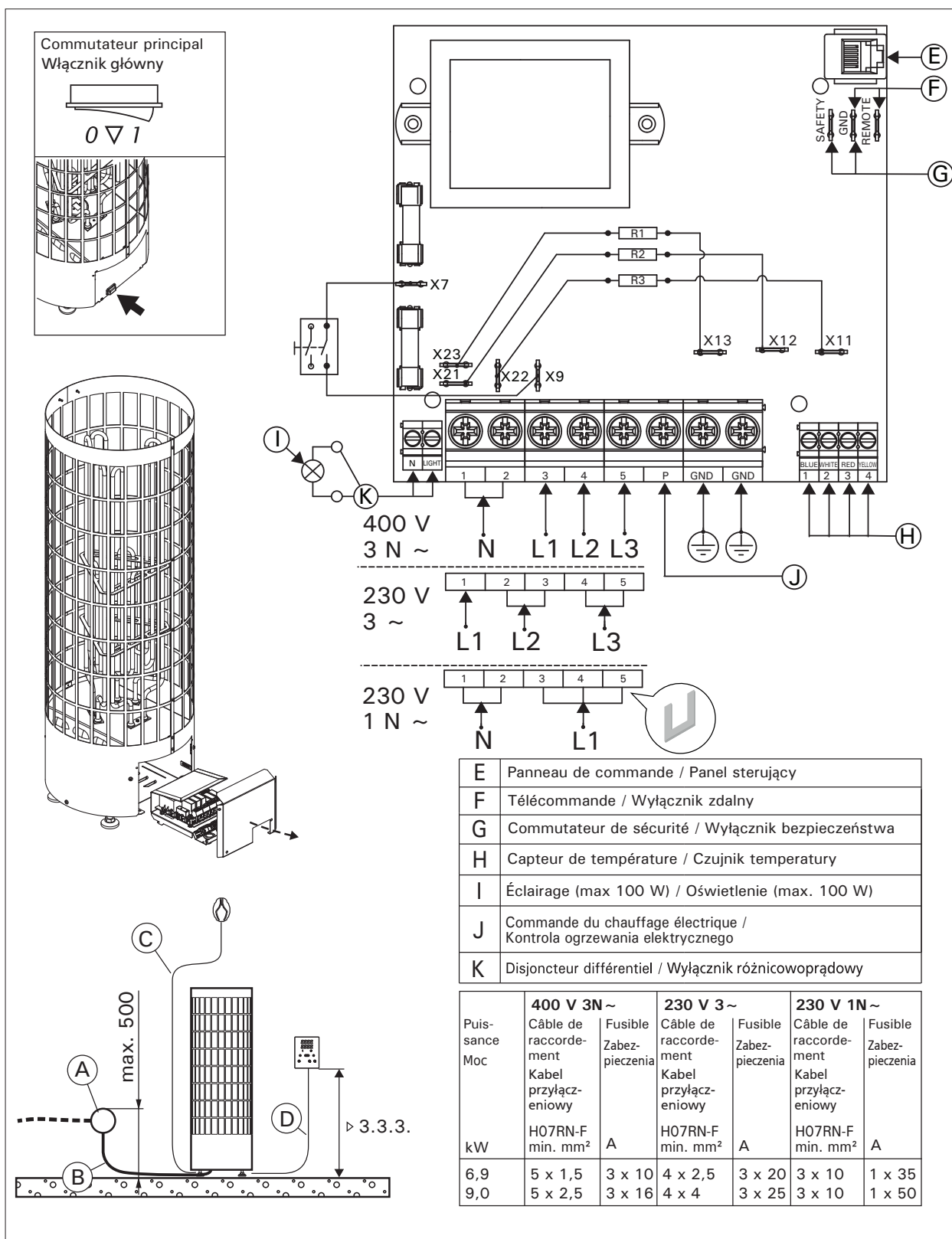
Figure 7. Raccordement électrique Rys. 7. Podłączenie elektryczne
