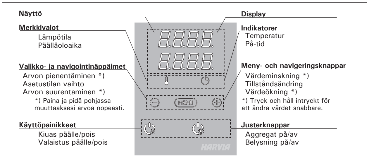
Kuva 2. Ohjauspaneeli Bild 2. Styrpanel
