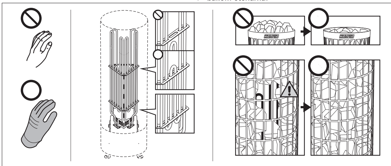
Kuva 1. Kiuaskivien latominen Bild 1. Stapling av bastustenar
