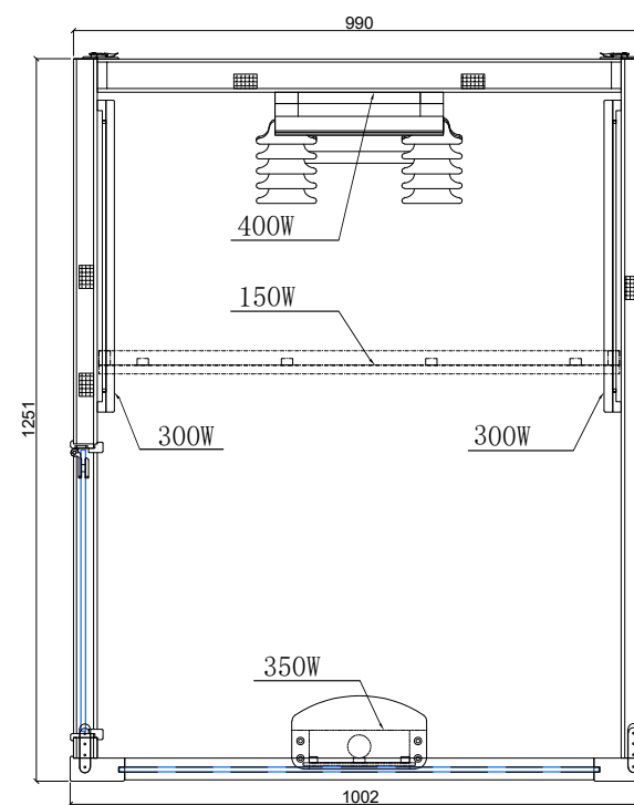
Draufsicht
