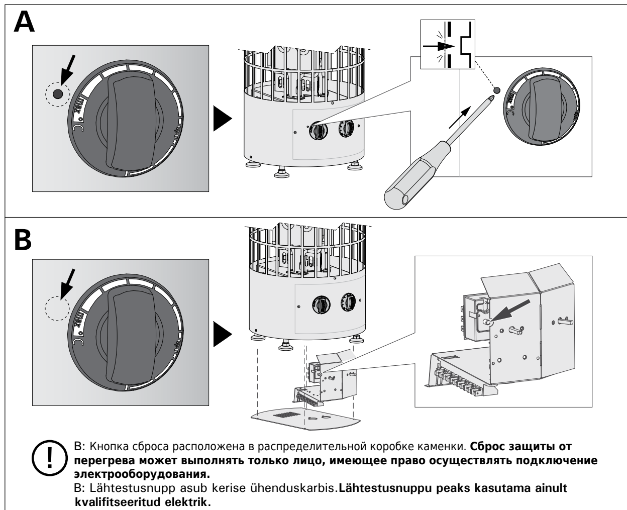
Рисунок 10. Кнопка сброса защиты от перегрева
