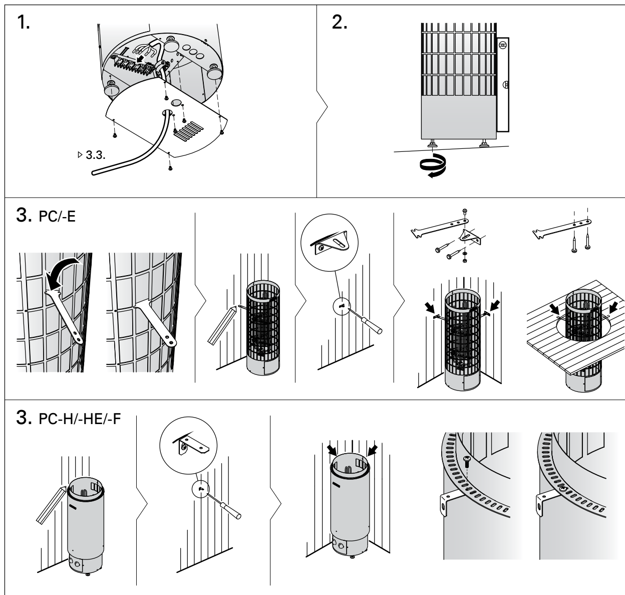
Рисунок 9. Установка каменки
