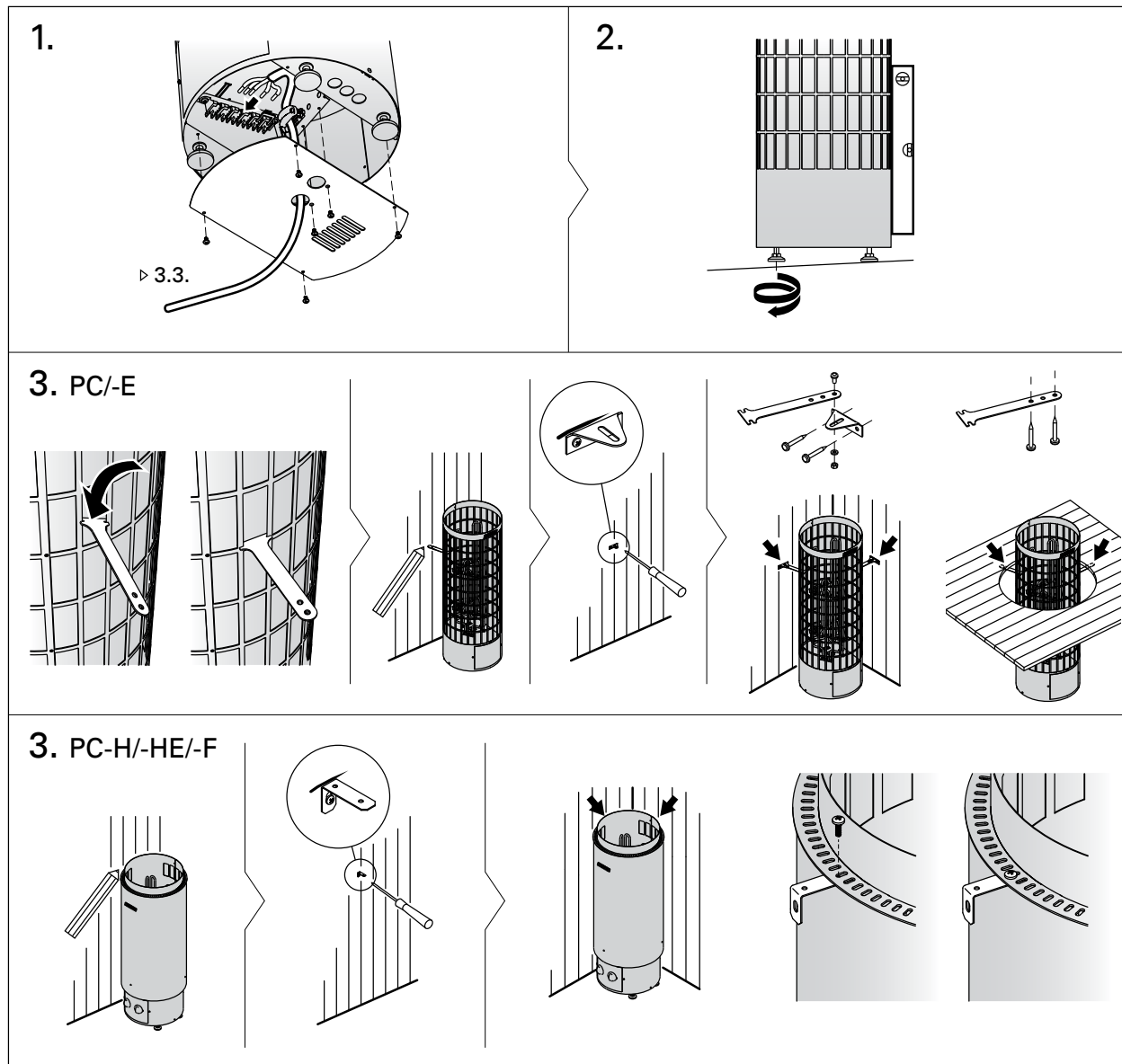
Kuva 9. Kiukaan asentaminen Bild 9. Montering av aggregatet
