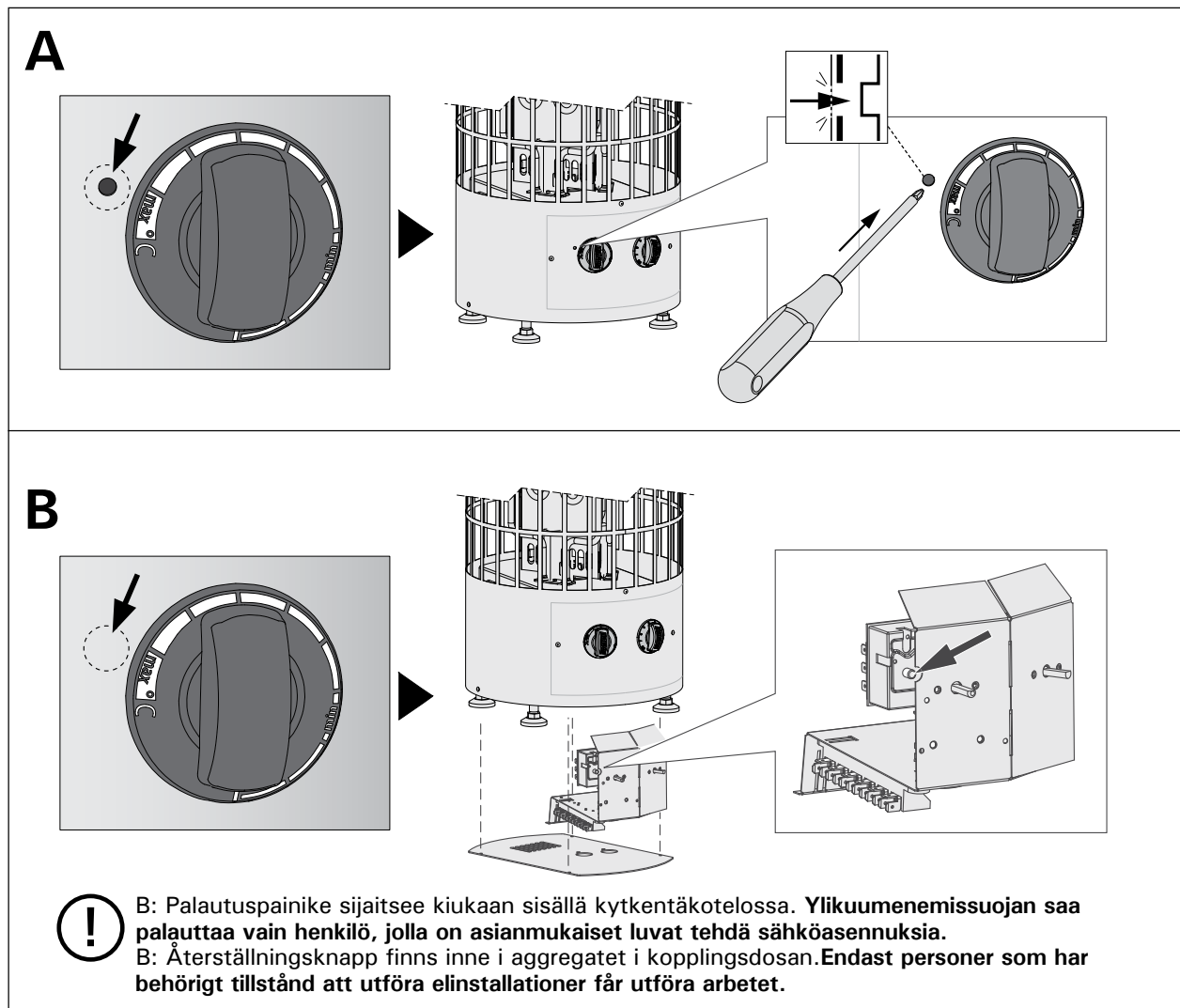
Kuva 10. Ylikuumenemissuojan palautuspainike
