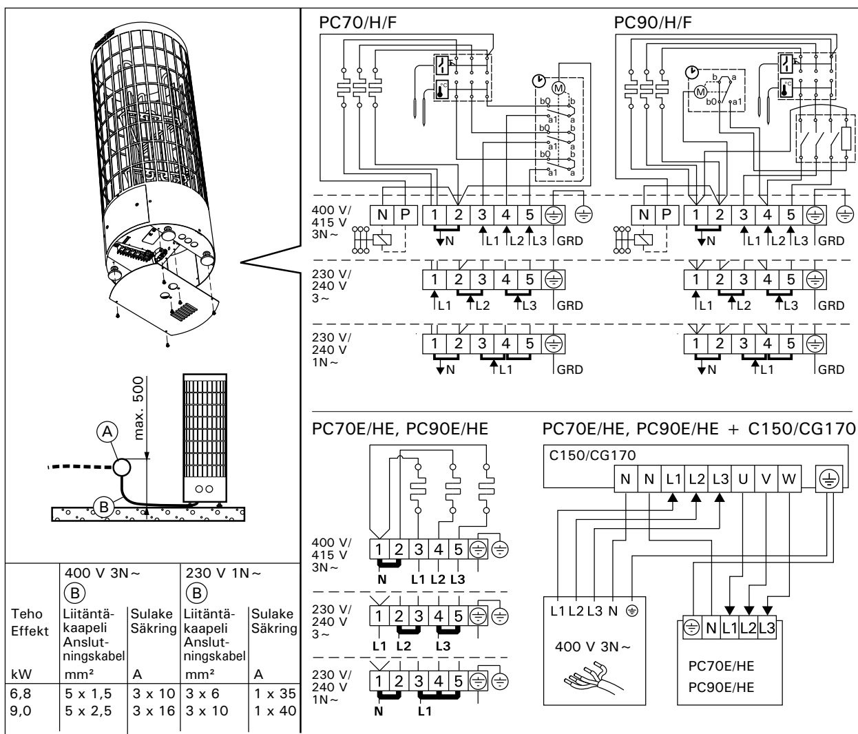
Kuva 7. Sähkökytkennät Bild 7. Elinstallationer
