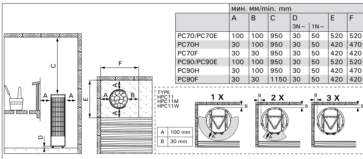
Рисунок 6. Расположение и безопасные расстояния (все размеры приведены в миллиметрах) Joonis 6. Ohutuskaugused (kõik mõõtmised millimeetrites)
