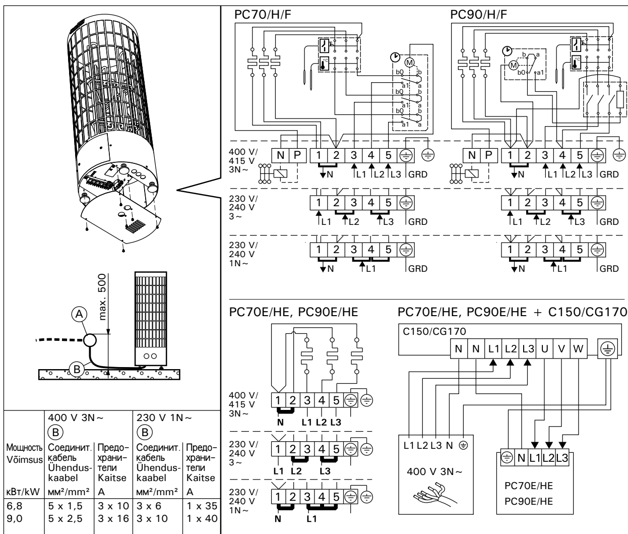
Рисунок 7. Электромонтаж Joonis 7. Elektrihendused
