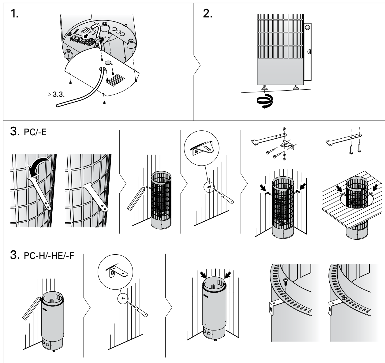
Figure 9. Installing the heater Abbildung 9. Installation des Saunaofens
